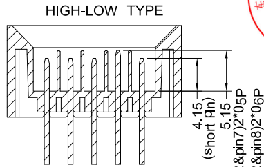
SECTION A-A SCALE:1:1
