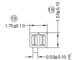
SECTION D-D SCALE 1:1
