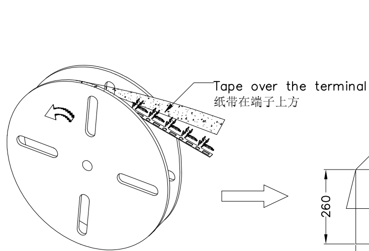
卷装方式 Package way
