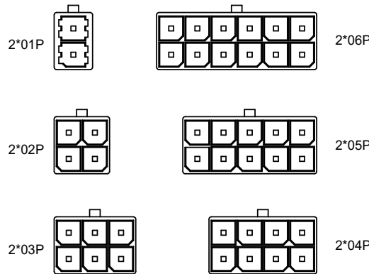
2*01P~2*06P 视图
