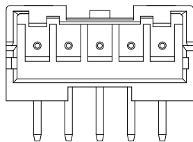
5Pin
